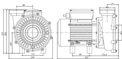
SOLUBLOC #10 (0,4 kW)
