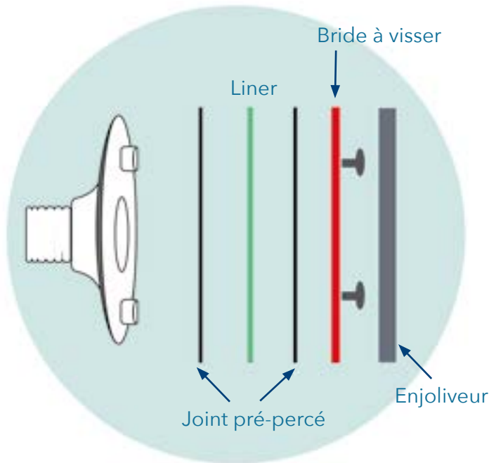
Ordre de montage de l'étanchéité d'une pièce à sceller
