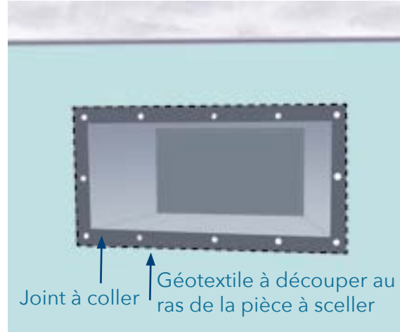
Ordre de montage de l'étanchéité d'une pièce à sceller
